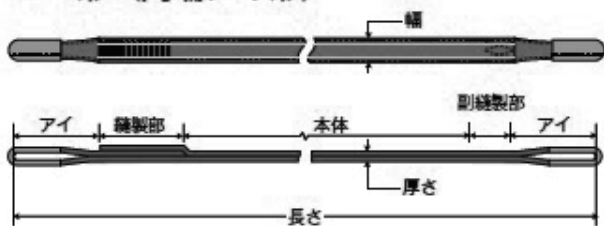
IV E 形（両端アイ形）
